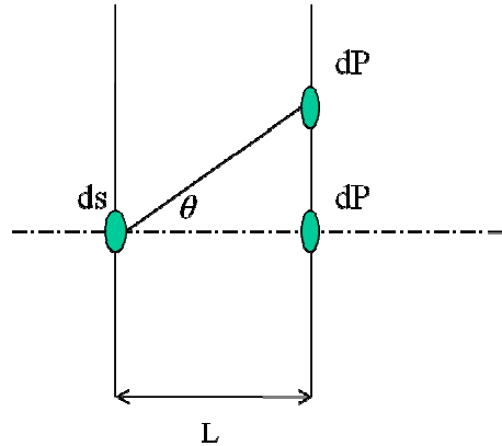
図4 向かい合う平面上の照度
